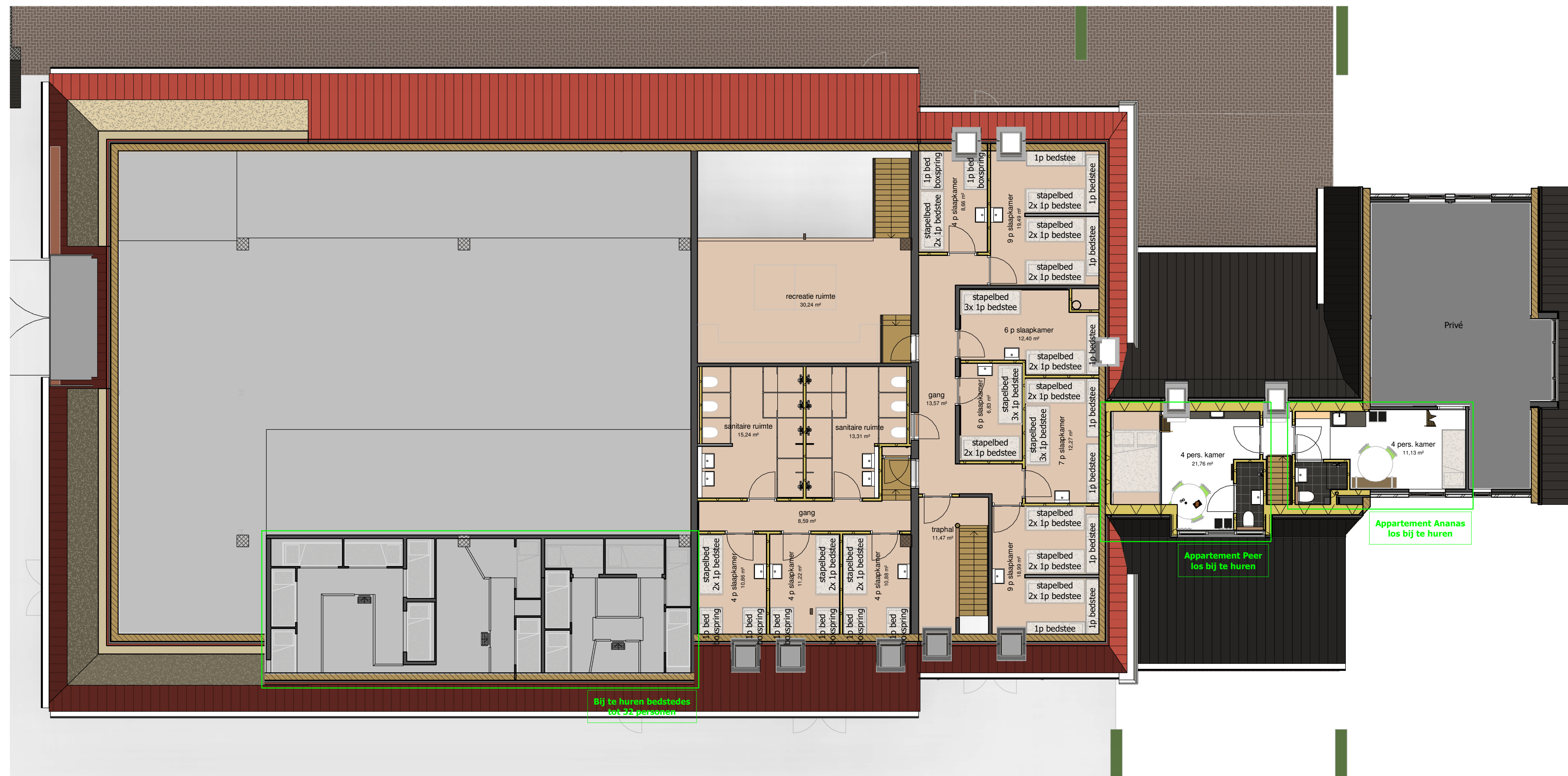
eerste verdieping 1 : 100
